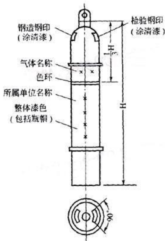
图 4-3 气瓶的颜色标记喷涂位置
